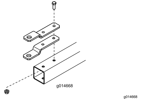
图 8 高挂钩位置
