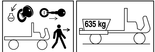
ANTES DE ABANDONAR EL ASIENTO QUITA EL CONTACTO Y RETIRA LA LLAVE CARGA NOMINAL, TOLVA
