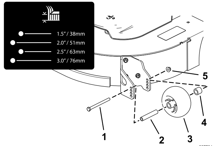
Figura 27 Máquinas de descarga lateral
