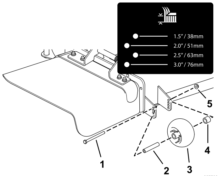
Figura 26 Máquinas de descarga lateral
