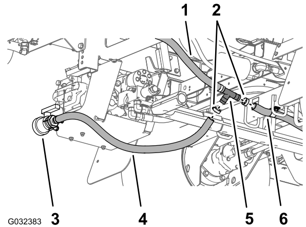
Figura 42 Máquinas de 2016
