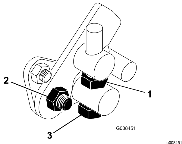
1. Контргайка
