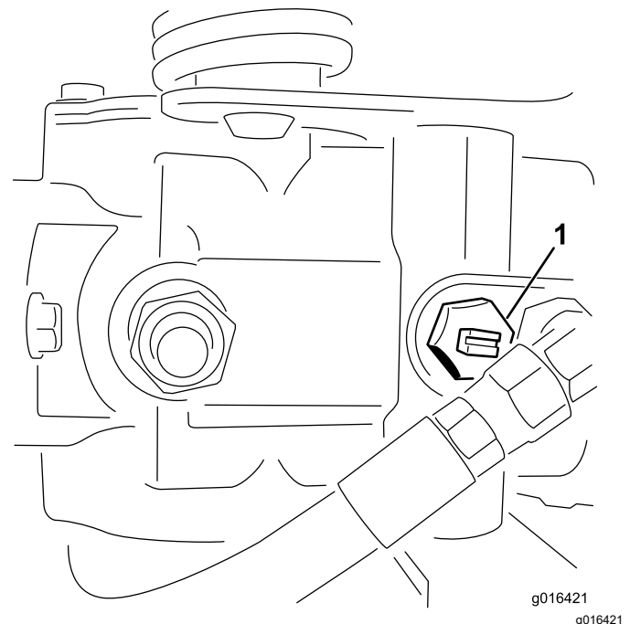
Figuur 24 Onderaanzicht
