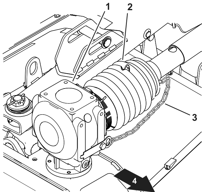
Рисунок 21 Кожух приводного вала правой деки
