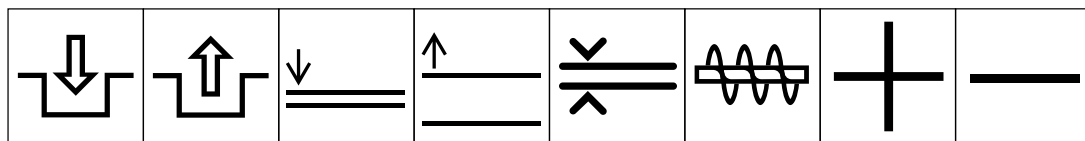
Embragar Desembragar Bajar accesorio Subir accesorio Distancia de espaciamiento Quitanieves, barrena colectora Más/aumento/ polaridad positiva Menos/dismin- uación/polaridad negativa
