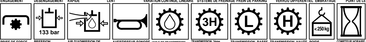
PRISE DE FORCE PRESSION HYDRAULIQUE AIR D'ADMISSION DE PRESSION HYDRAULIQUE AVERTISSEUR SONORE HUILE DE TRANSMISSION TRANSMISSION, 3ème RAPPORT HAUT TRANSMISSION, BASSE TRANSMISSION, HAUTE POIDS COMPTEUR HORAIRE - HEURES D'UTILISATION
