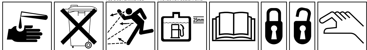
LIQUIDES CAUSTIQUES, BRULURES CHIMIQUES DES DOIGTS OU DE LA MAIN NE PAS JETER A LA POUBELLE PROJECTION D'OBJETS - EXPOSITION DE TOUT LE CORPS REPERE DE REMPLISSAGE DU RESERVOIR LIRE LA NOTICE D'UTILISATION VERROUILLAGE DEVERROUILLAGE MANUEL
