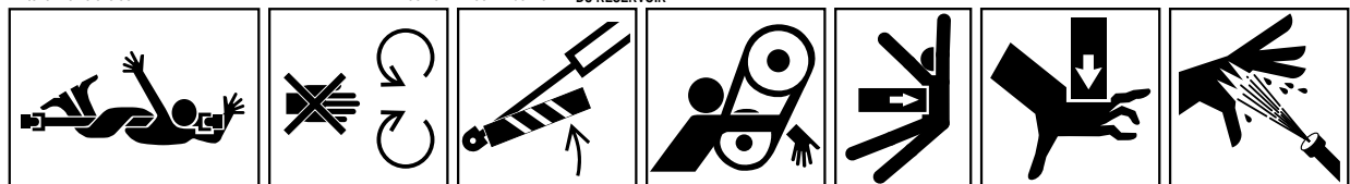
HAPPEMENT DE TOUT LE CORPS - TRANSMISSION D'ENTREE DE L'ACCESSOIRE NE PAS OUVRIIR OU ENLEVER LES CAPOTS DE SECURITE QUAND LE MOTEUR TOURNE BLOQUER LE VERIN DE LEVAGE AVEC LE DISPOSITIF APPROPRIE AVANT D'ABORDER UNE ZONE DANGEREUSE HAPPEMENT DE LA MAIN & DU BRAS - CHAINE DE TRANSMISSION ECRASEMENT LATERAL DU TORSE ECRASEMENT DES DOIGTS OU DE LA MAIN PAR LE HAUT CICLEUR HAUTE PRESSION - EROSION DE LA CHAIR
