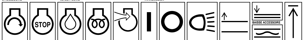
DEMARRAGE DU MOTEUR ARRRET DU MOTEUR HUILE DE GRAISSAGE DU MOTEUR BOUGIE DE PRECHAUFFAGE ADMISSION D'AIR DE COMBUSTION DU MOTEUR CONTACT/ MARCHÉ CONTACT COUPE/ ARRÉT PHARES RELEVAGE ACCESSOIRE FLOTTATION ACCESSOIRE MOUVEMENT RECTILIGNE LIMITE
