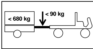
CHARGE NOMINALE - REMORQUE ET FLECHE
