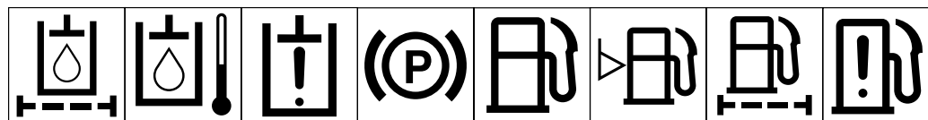
Filtere d'huile hydraulique Température d'huile hydraulique Défaillance/panne de circuit d'huile hydraulique Frein de parking Carburant Niveau de carburant Filtere à carburant Défaillance/panne de circuit d'alimentation
