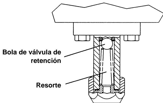
BOQUILLA ABIERTA
