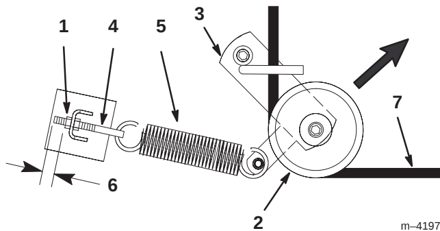
Figuur 43 Bovenaanzicht
