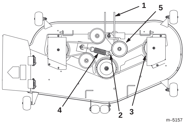
Figuur 44 Bovenaanzicht
