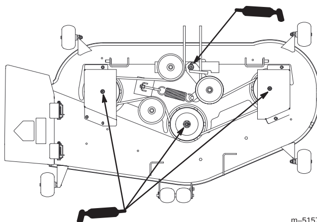
Figuur 30 Bovenaanzicht
