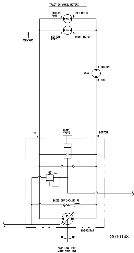
Hydraulikaavio (Rev. B)
