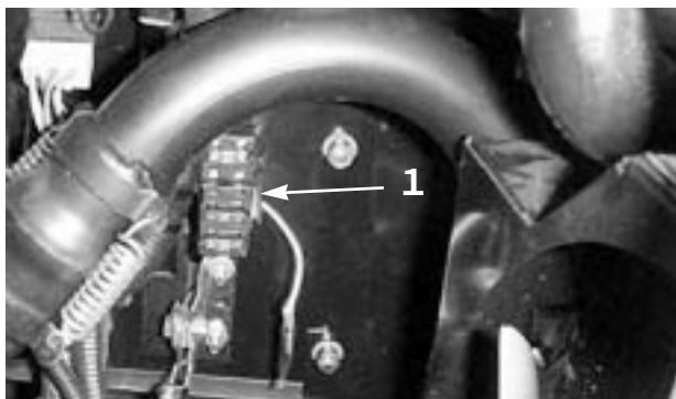
図 63 1. ヒューズ
