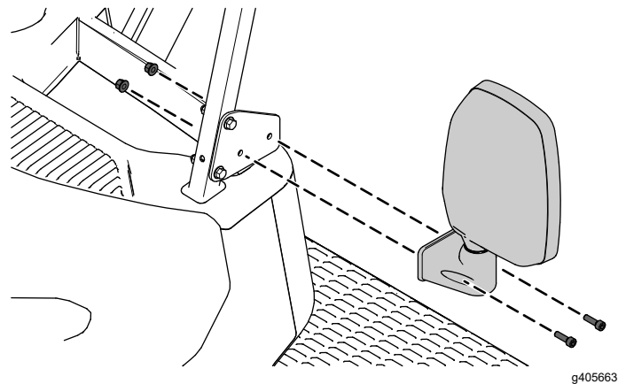
Figuur 4 Installatie onderaan links getoond
