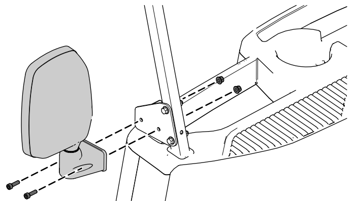
Figuur 5 Installatie onderaan rechts getoond
