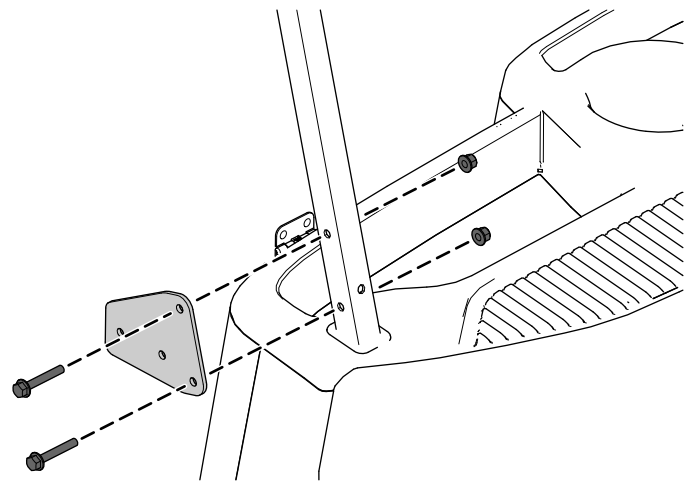
Figuur 3 Installatie onderaan rechts getoond
