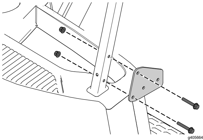
Figuur 2 Installatie onderaan links getoond
