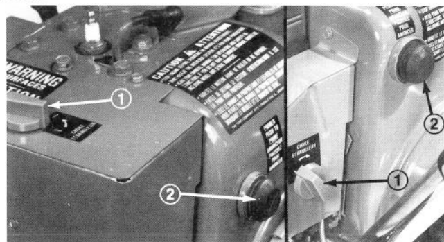
Déneigeuse 624
