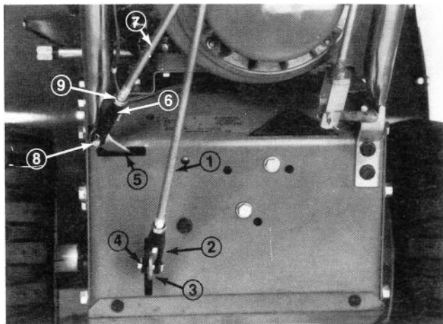
Déneigeuse 824 Figure 6
