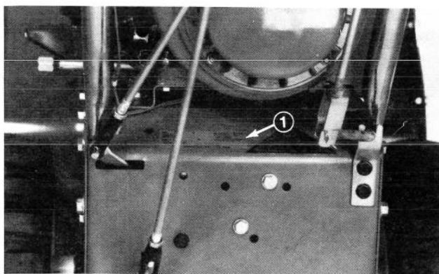
Déneigeuse 824 Figure 39
