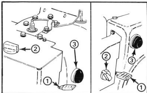
Déneigeuse 624 Déneigeuses 824 et 828
