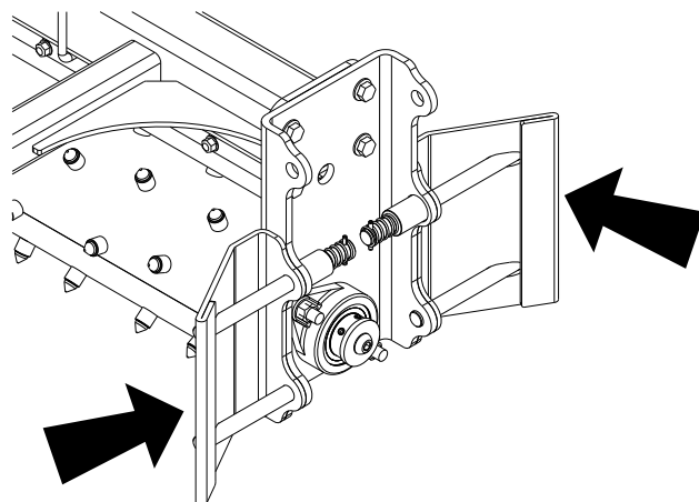
Figuur 4 Werkstand
