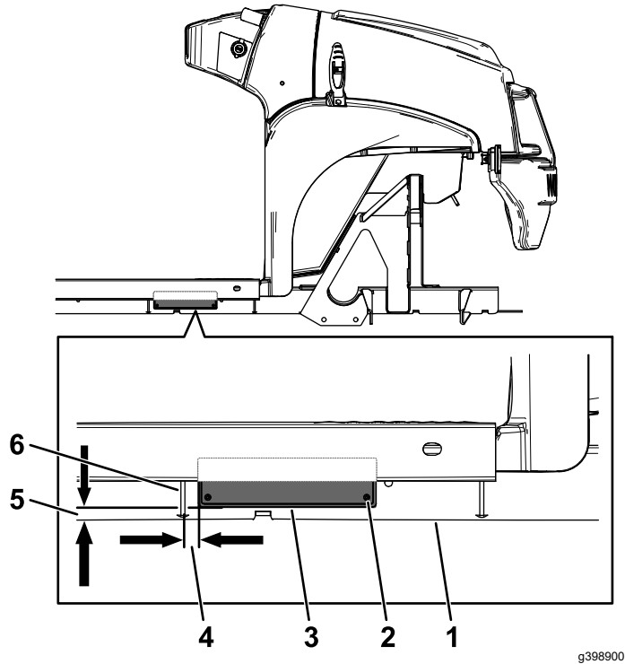
图 6 1. 机架 4. 11mm 2. 弹伸铆钉 (3 x 10mm) 5. 11mm 3. 序列号牌 6. 支持
