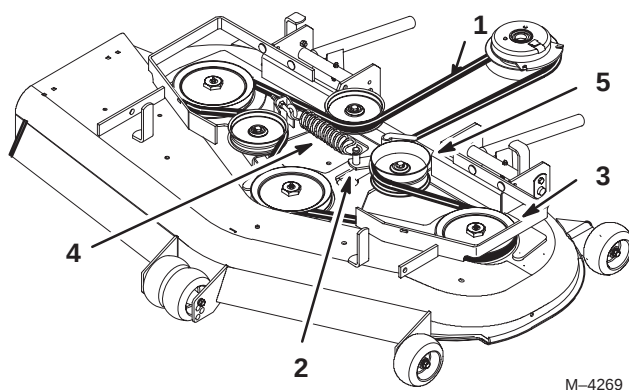
Figuur 67 Bovenaanzicht
