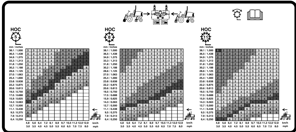
図 55 5" 127 mm リールの速度表
