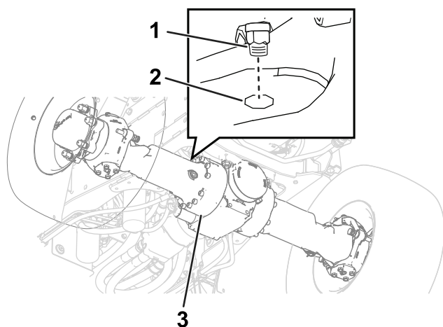
Figura 103 Eje Delantero
