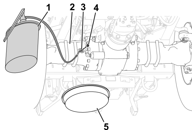
Figura 102 Eje trasero
