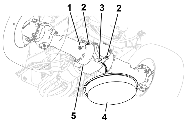
Figura 99 Eje Delantero
