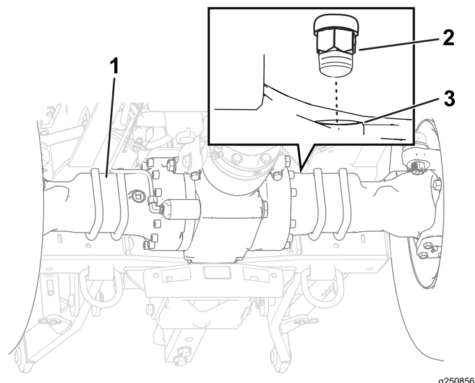
Figura 104 Eje trasero
