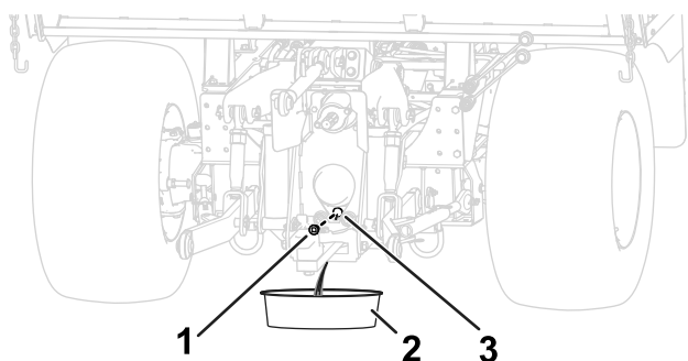
Figura 100 Eje trasero
