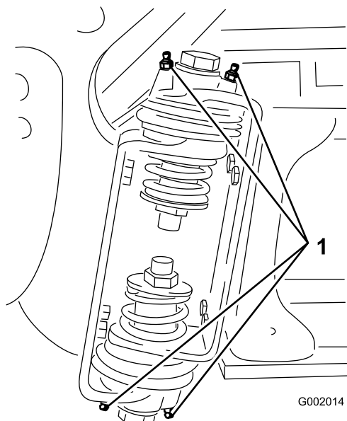
図 102 右ブーム
