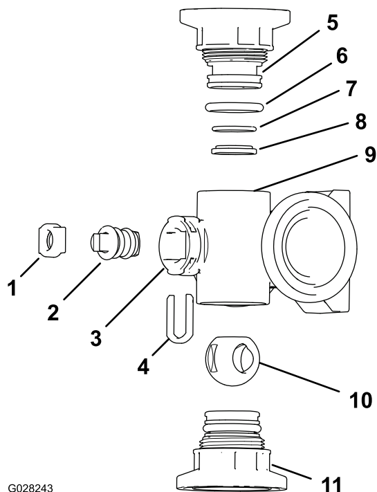
图 129 搅拌阀歧管
