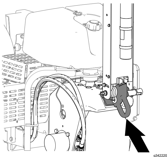
Рисунок 135 Передняя скоба
