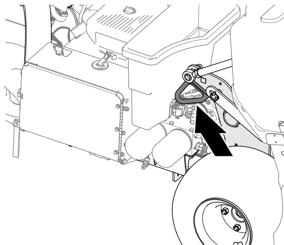
Рисунок 137 Левая задняя скоба
