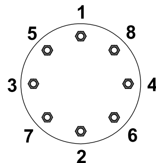
Figur 18 Framhjul
