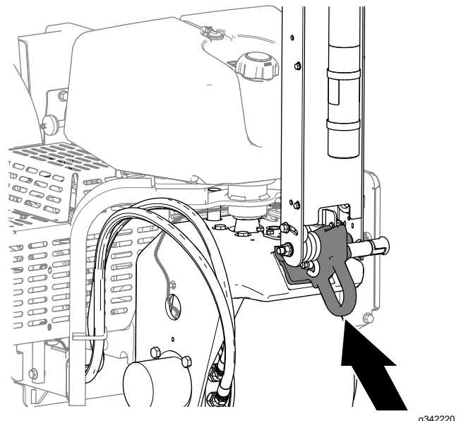
Figura 135 Anclaje delantero
