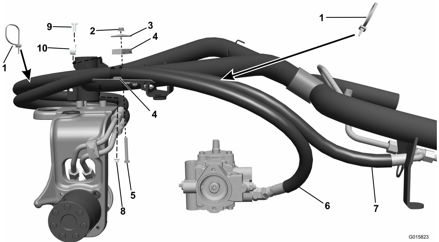
Figur 10 Dieselmotor
