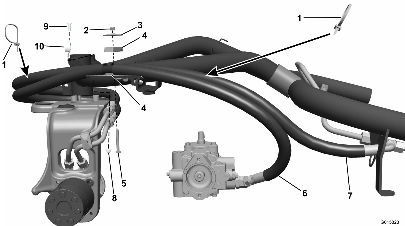
Figuur 10 Dieselmotor
