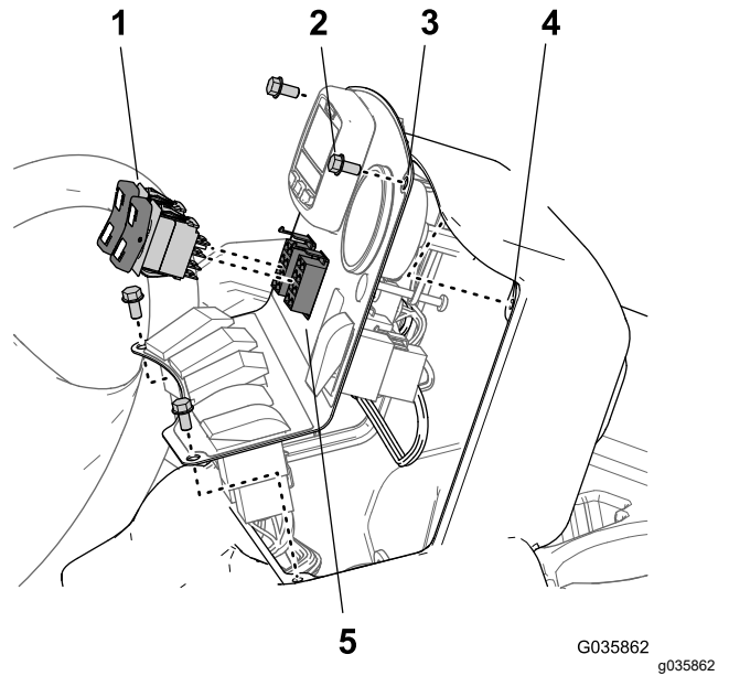
그림 37 Multi Pro WM 장비
