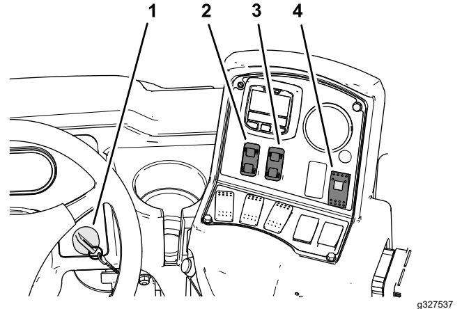
그림 42 Multi Pro WM 장비
