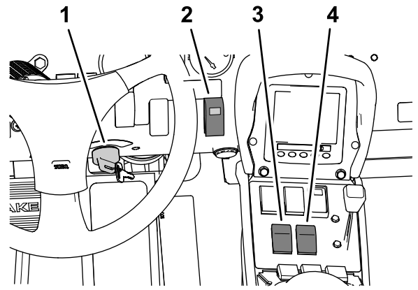
그림 41 Multi Pro 5800 장비
