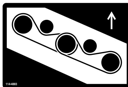
Figuur 131 Linkermaaidek
