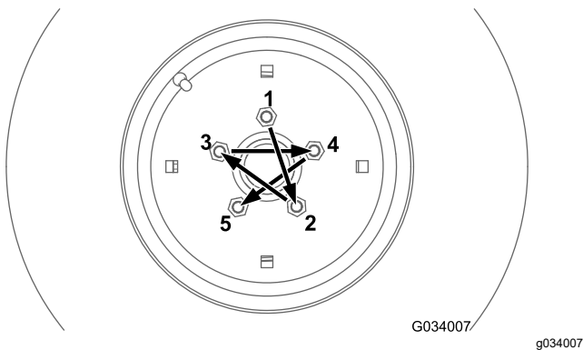
Bild 57 Vorderrad
