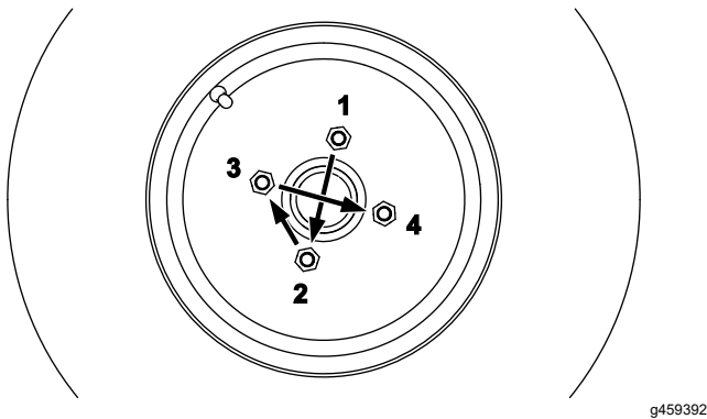
Bild 58 Hinterrad
