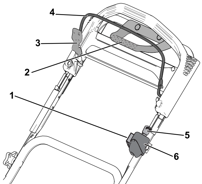
Figur 8 Övre handtag
