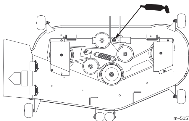
Figura 31 Vista Superior
