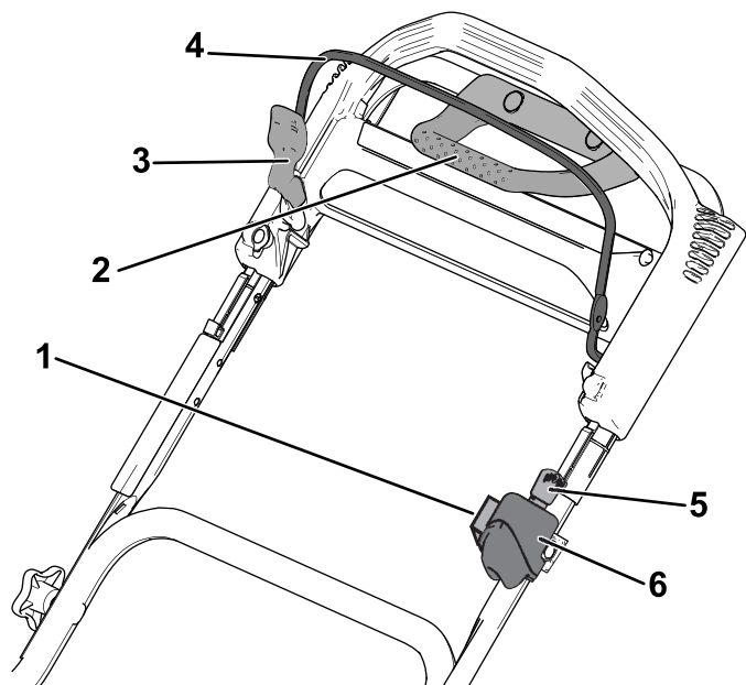
Slika 8 Gornja ručka
