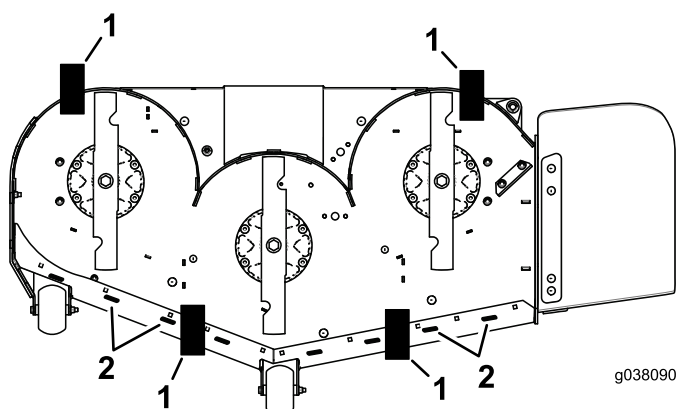
Figuur 84 Onderaanzicht
