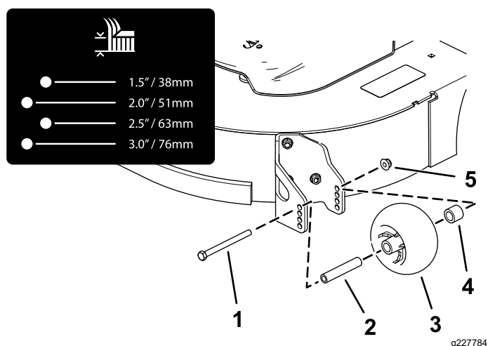
Figuur 28 Machines met zijafvoer
