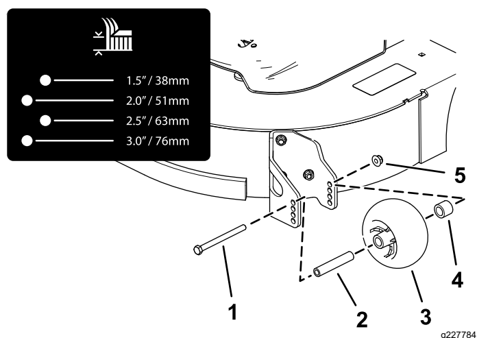
Figur 28 Maskiner med sideudkast
