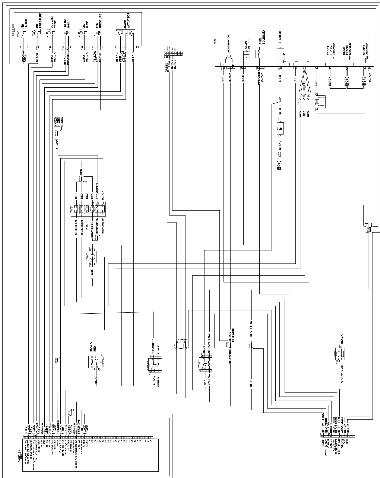
Електрична схема - двигун Yanmar 3TNV80FT (Rev. B)
