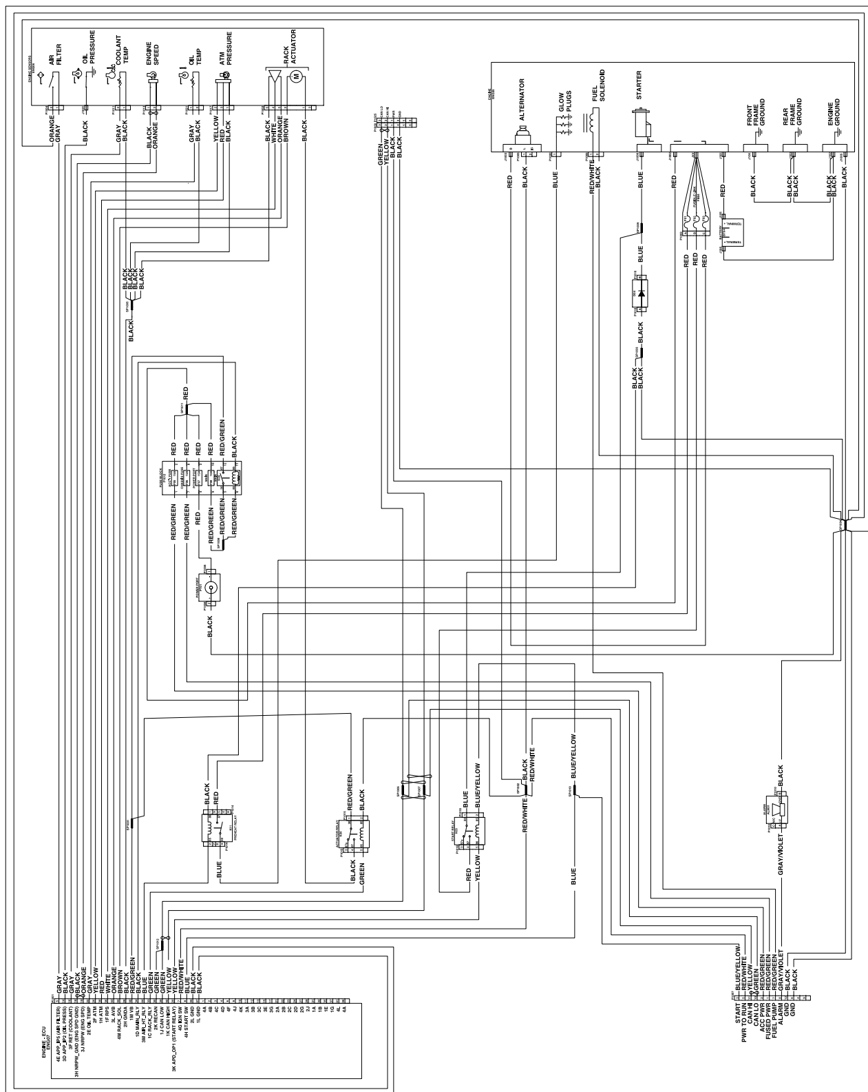
Elektriskt kopplingsschema – Yanmar-motor 3TNV80FT (Rev. B)
