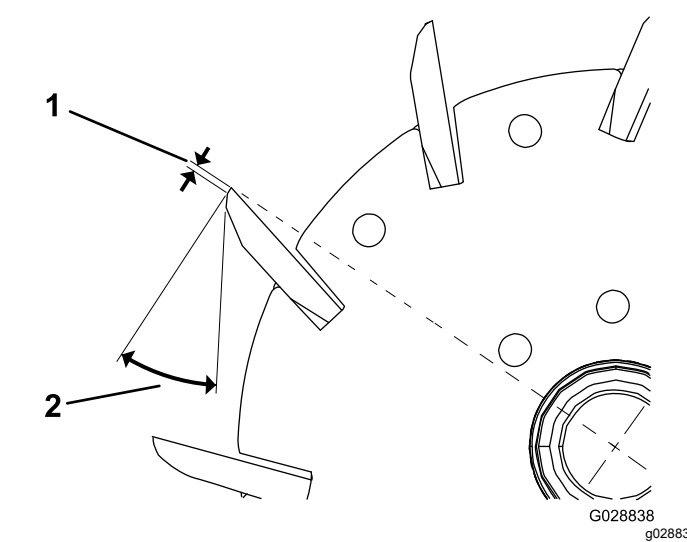
그림 35 전향 스위프형 릴
