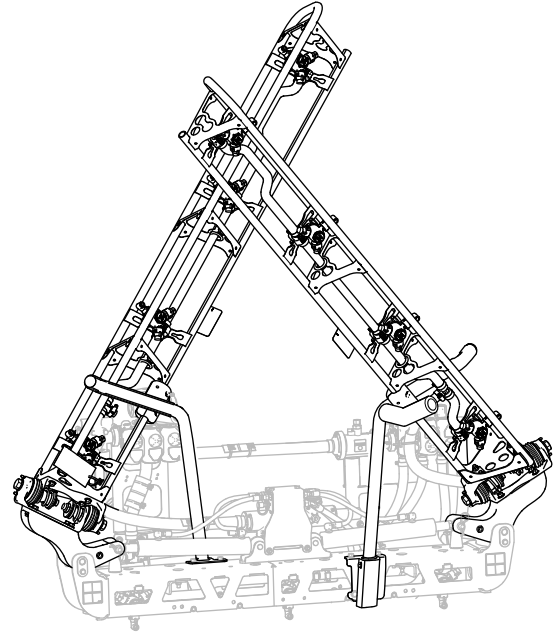
Şekil 26 "X" taşıma konumu
