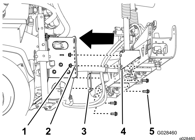
1. Kontranavrtka ( \frac{1}{2} " ) 2. Rupa 3 – odozdno (nosač strele) 3. Montažni nosač sekcije (levo) 4. Montažni nosač sekcije (desno) 5. Zavrtanj ( \frac{1}{2} x 1\frac{1}{4} " ) 3. Montirajte sklop srednje strele na ram platforme prskalice pomoću 4 zavrtnja ( \frac{1}{2} x 1\frac{1}{4} " ) i 4 navrtke ( \frac{1}{2} " ). 4. Zategnite zavrtnje i navrtke na 67 do 83 N·m.
