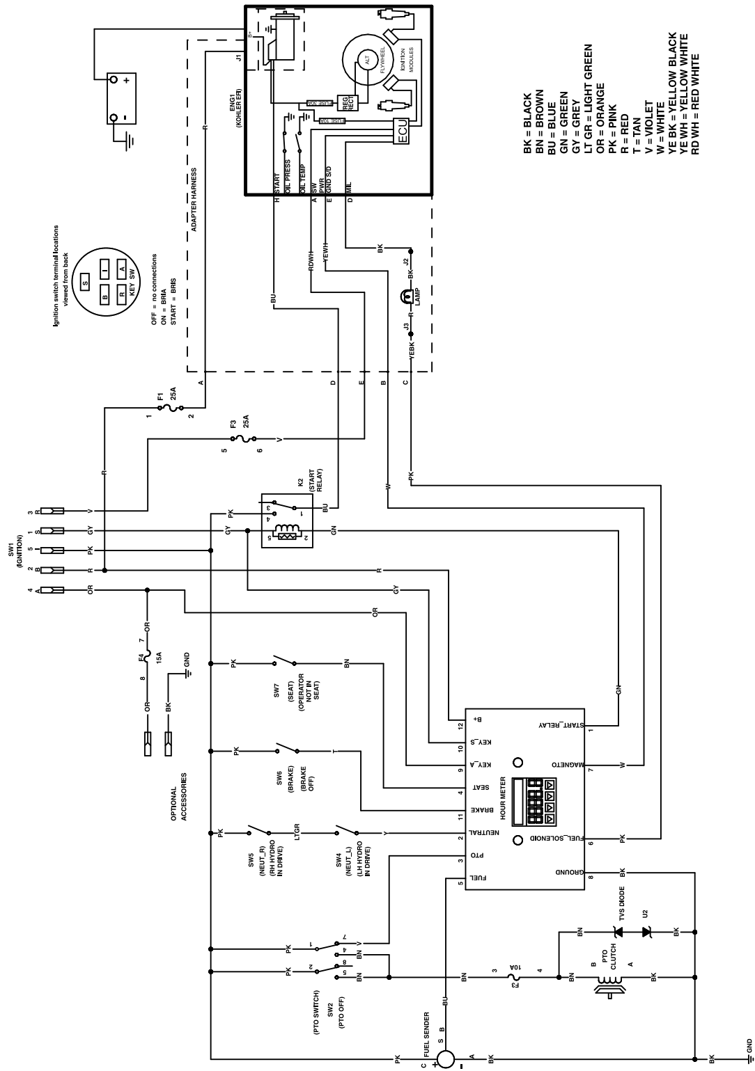
Schéma électrique (Rev. F)
