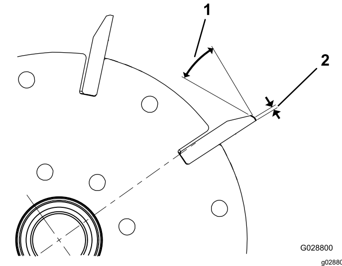
그림 34 레이디얼 릴
