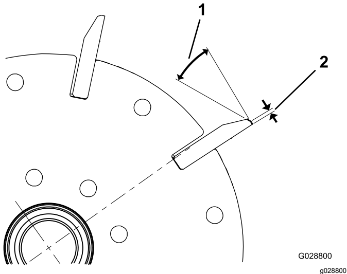
Rajah 34 Gelendong Jejari
