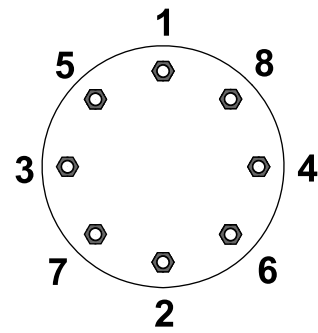
Figure 18 Roues avant
