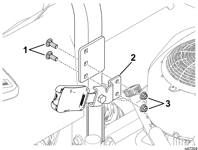
Figur 10 Spændeenhed vist
