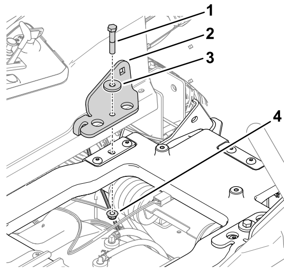
Figur 7 Sædeplatform vist
