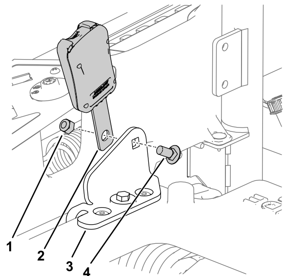
Figur 8 Spændeenhed vist. Gentag proceduren med trækstangenheden.
