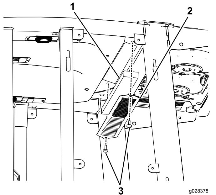
Bild 97 Interner Kabinenluftfilter
