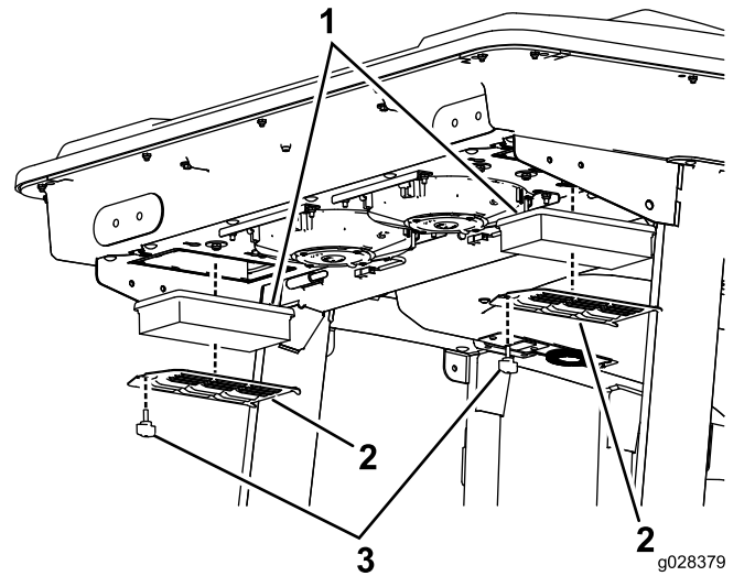
Bild 98 Hinterer Kabinenluftfilter
