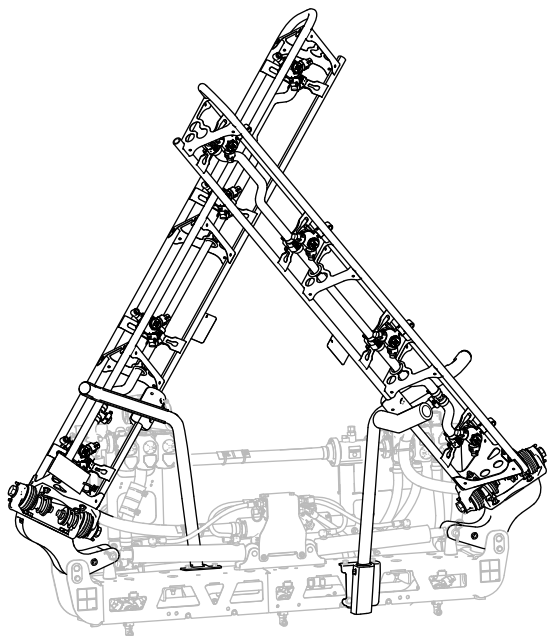
Kuva 51 X-kuljetusasento
